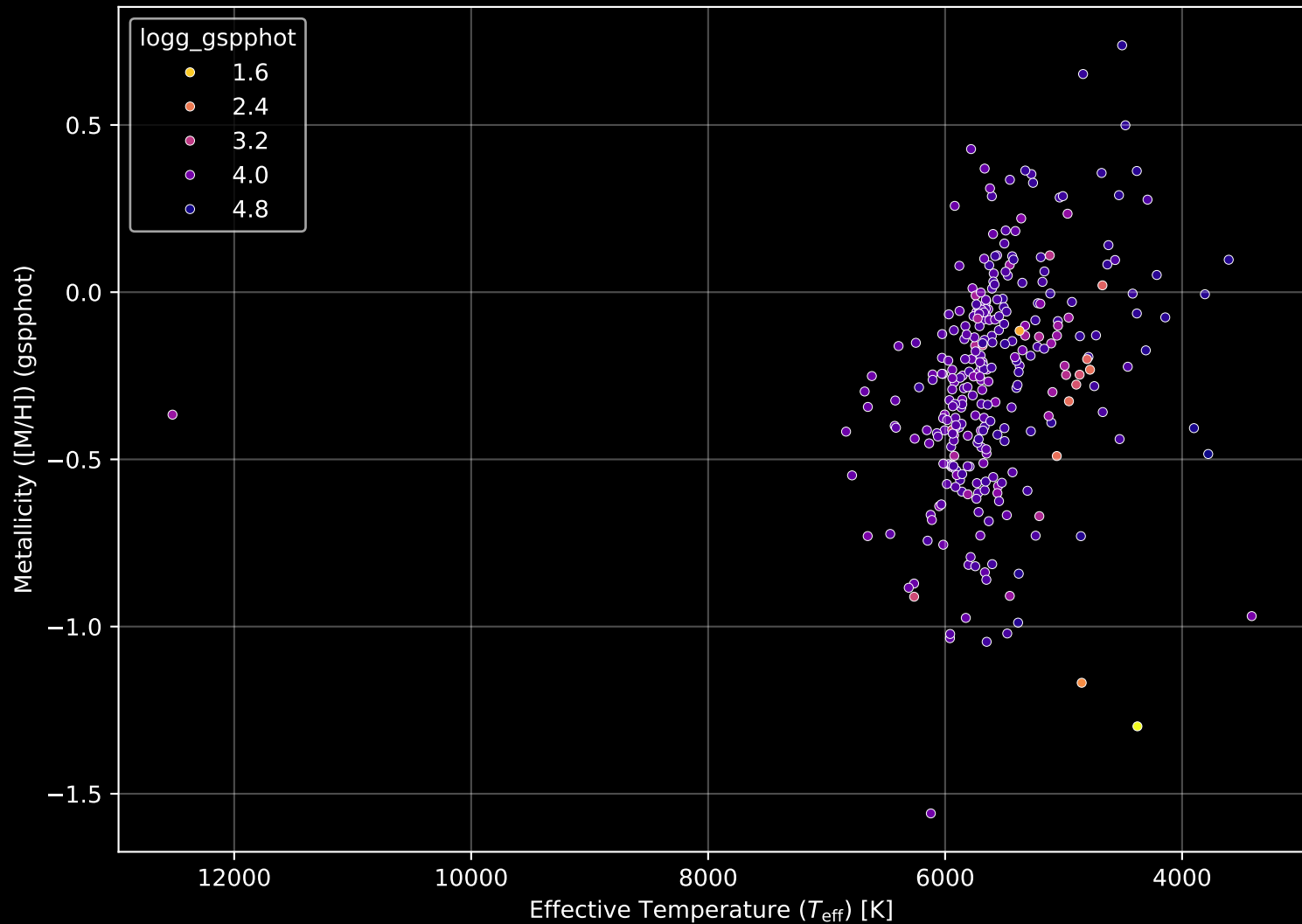
GALAH DR4 Field: [7010] Stellar Population Parameters (n= 300)
