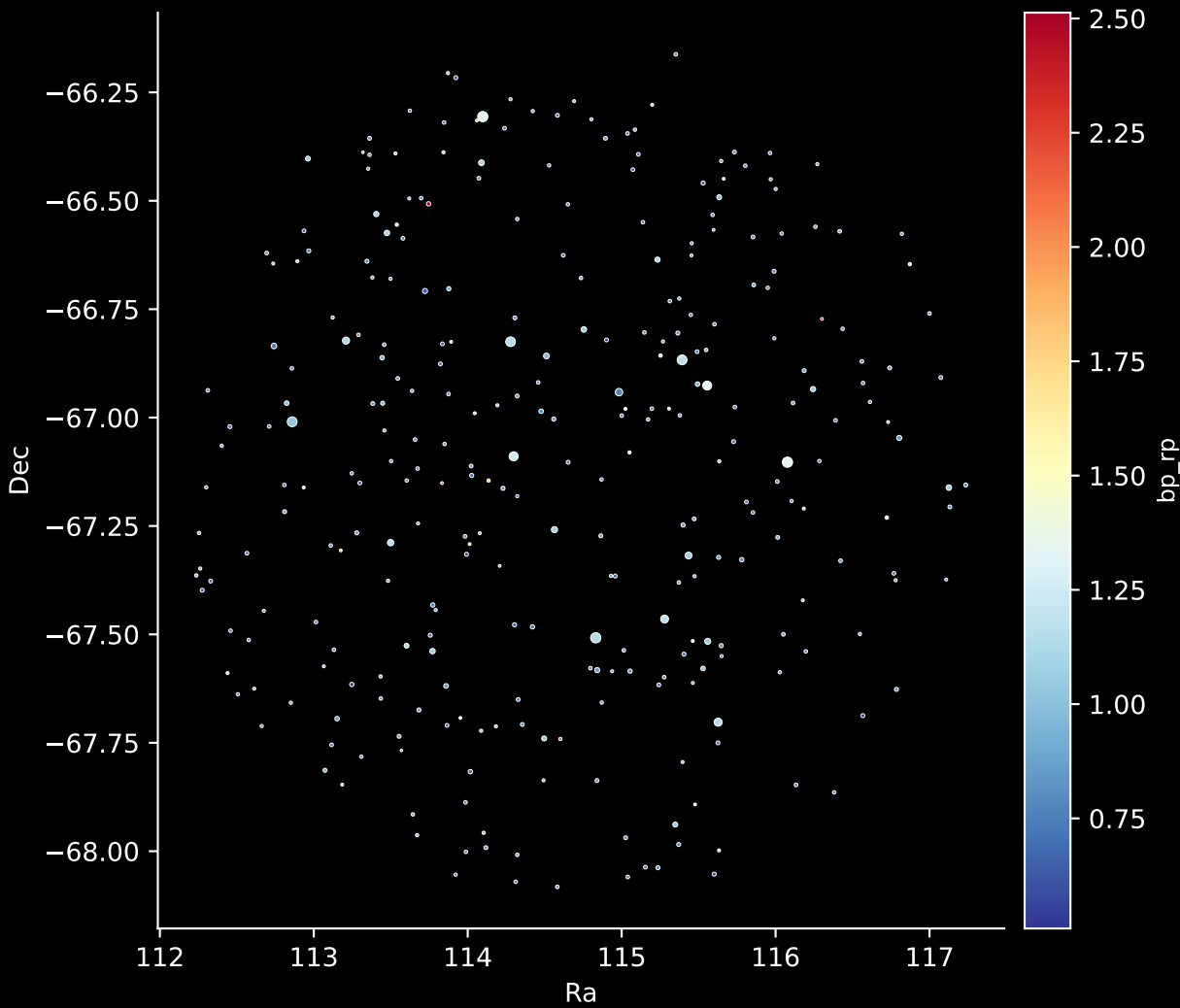
GALAH DR4 Field: [7010] Stars: 300
